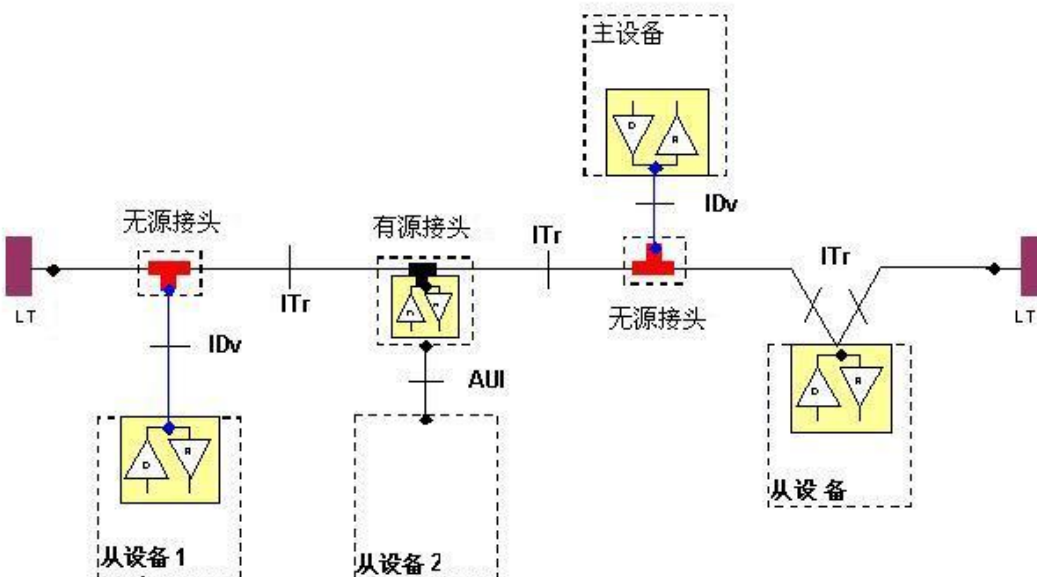
图 1 展现的是 MODBUS 多点串行链路系统中串行总线结构的总貌。
