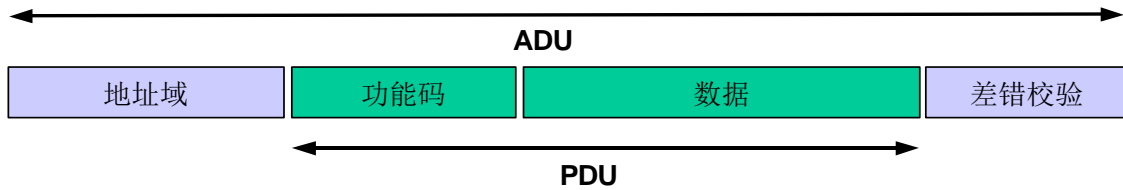
图 12：通用 MODBUS 帧
