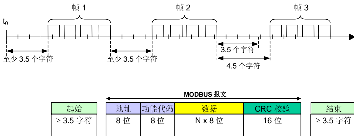
图 1: RTU 报文帧
