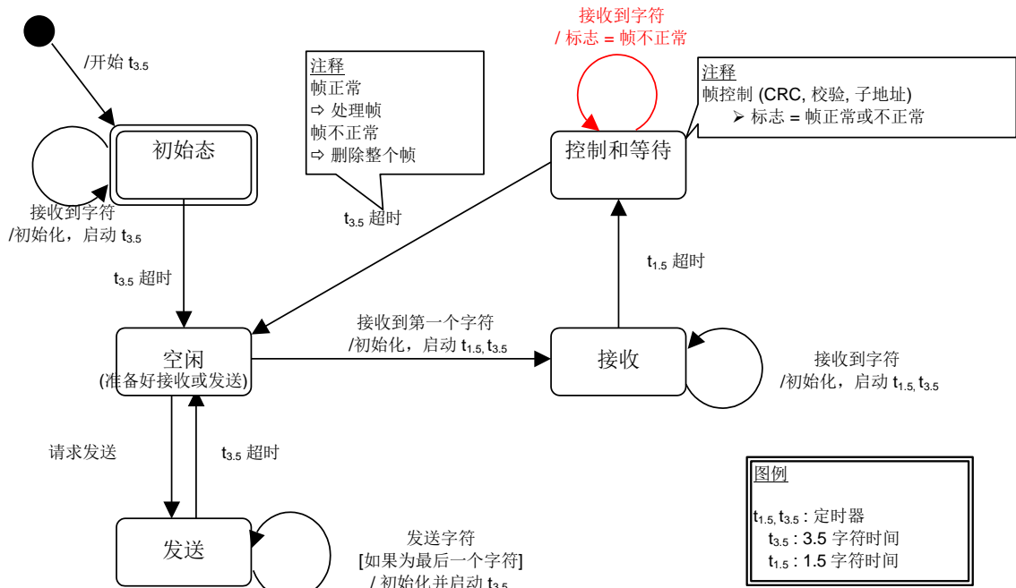
图 2: RTU 传输模式状态图
