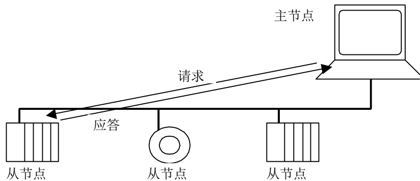
图 3： 单播模式
