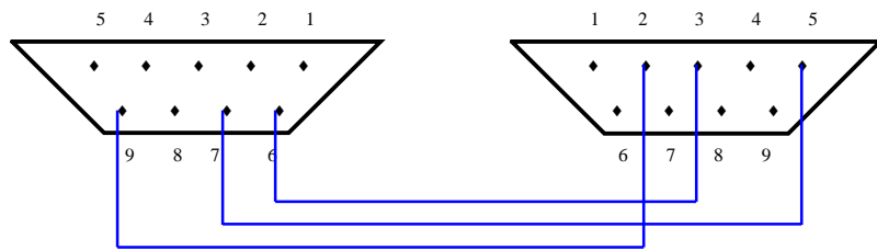
M2502 通讯电缆线
