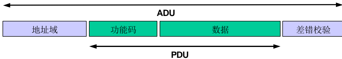
图 12: 通用 MODBUS 帧
