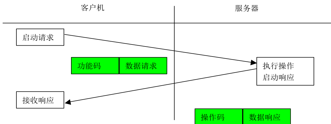
图 13: MODBUS 事务处理 (无差错)
