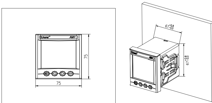
图 3 AMC72 安装尺寸
