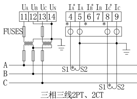
图9 仪表信号接线示意图
