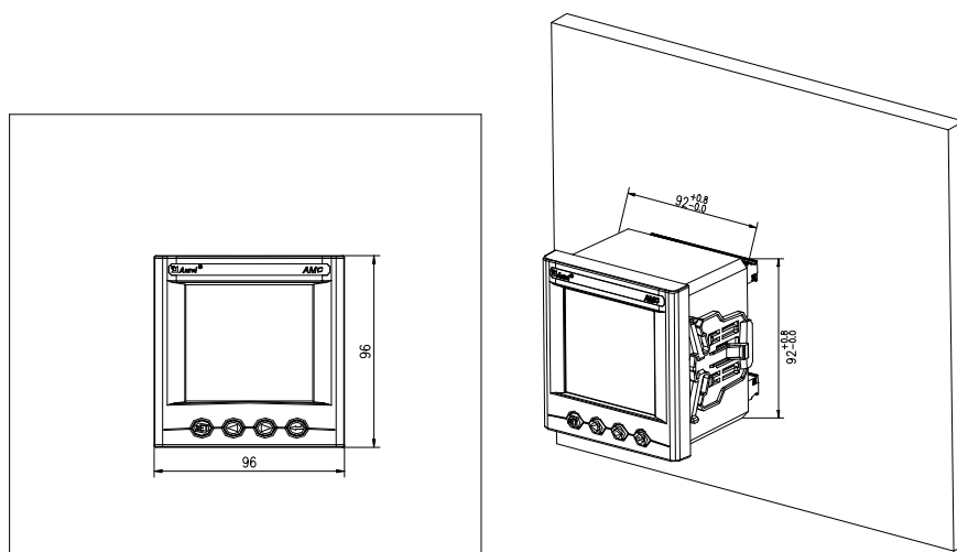
图 4 AMC96 安装尺寸
