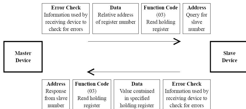
图 1-2 通讯流程
