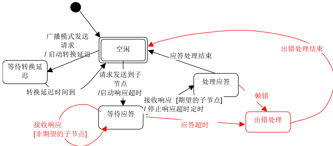
图 7： 主节点状态图
