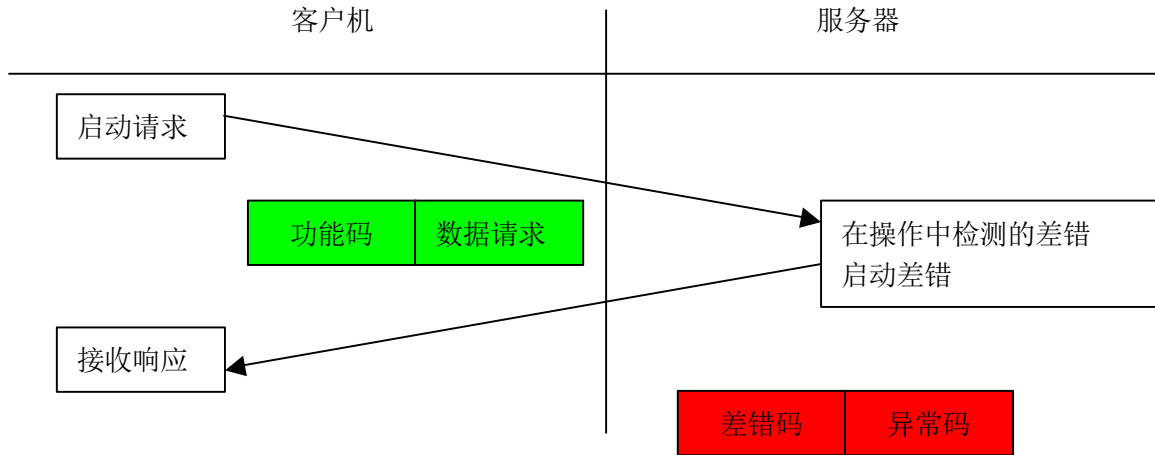
图 14 MODBUS 事务处理（异常响应）
