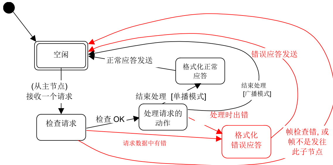
图 8：子节点状态图
