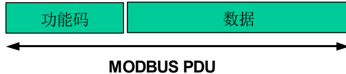
图 5: Modbus 协议数据单元
