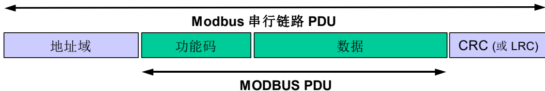
图 6: 串行链路上的 Modbus 帧
