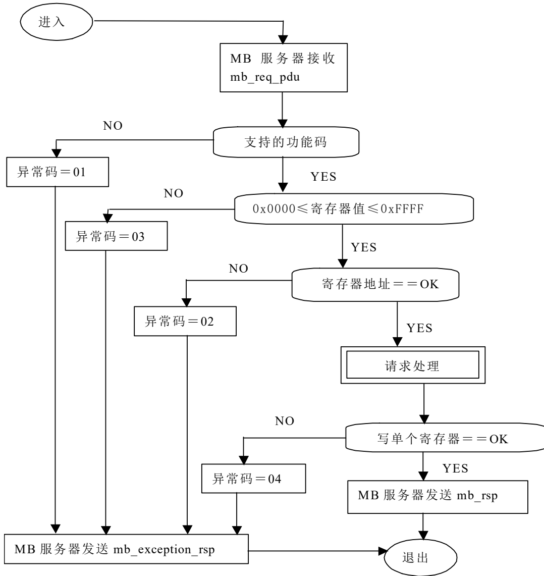
图 23: 写单个寄存器状态图
