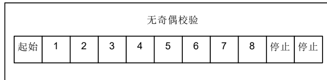
图 10: RTU 模式位序列(无校验的特殊情况)
