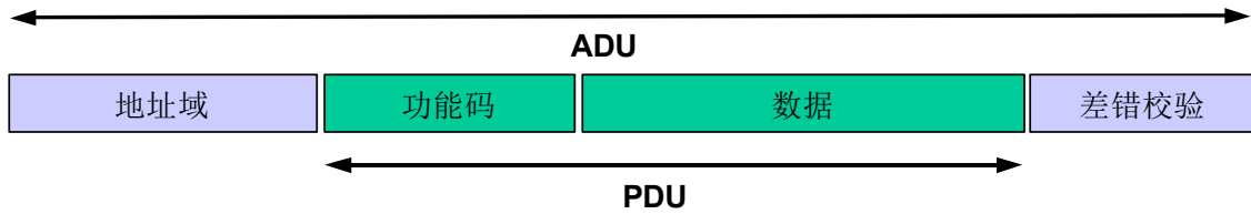
图 12: 通用 MODBUS 帧
