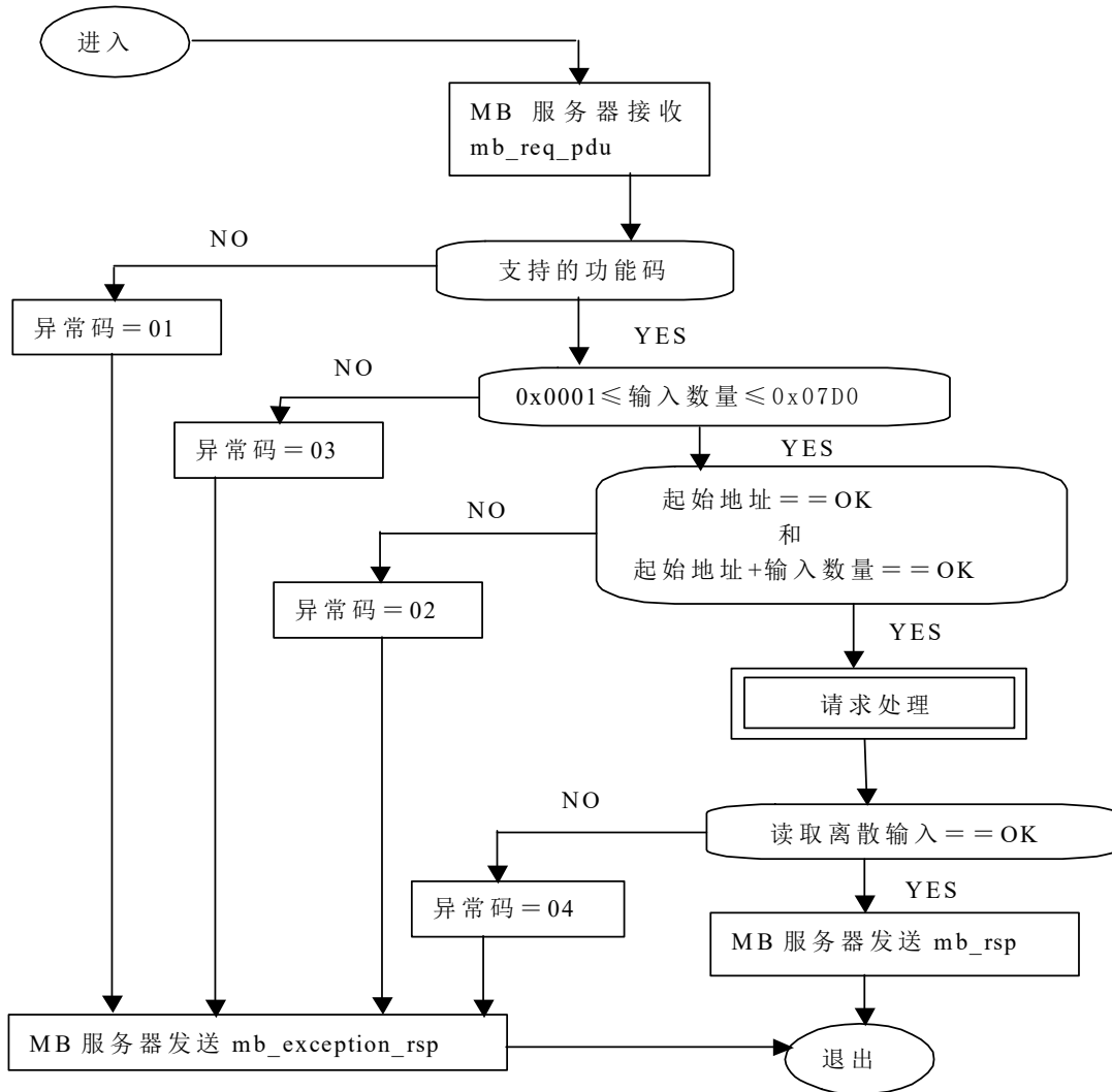
图 19: 读离散量输入的状态图
