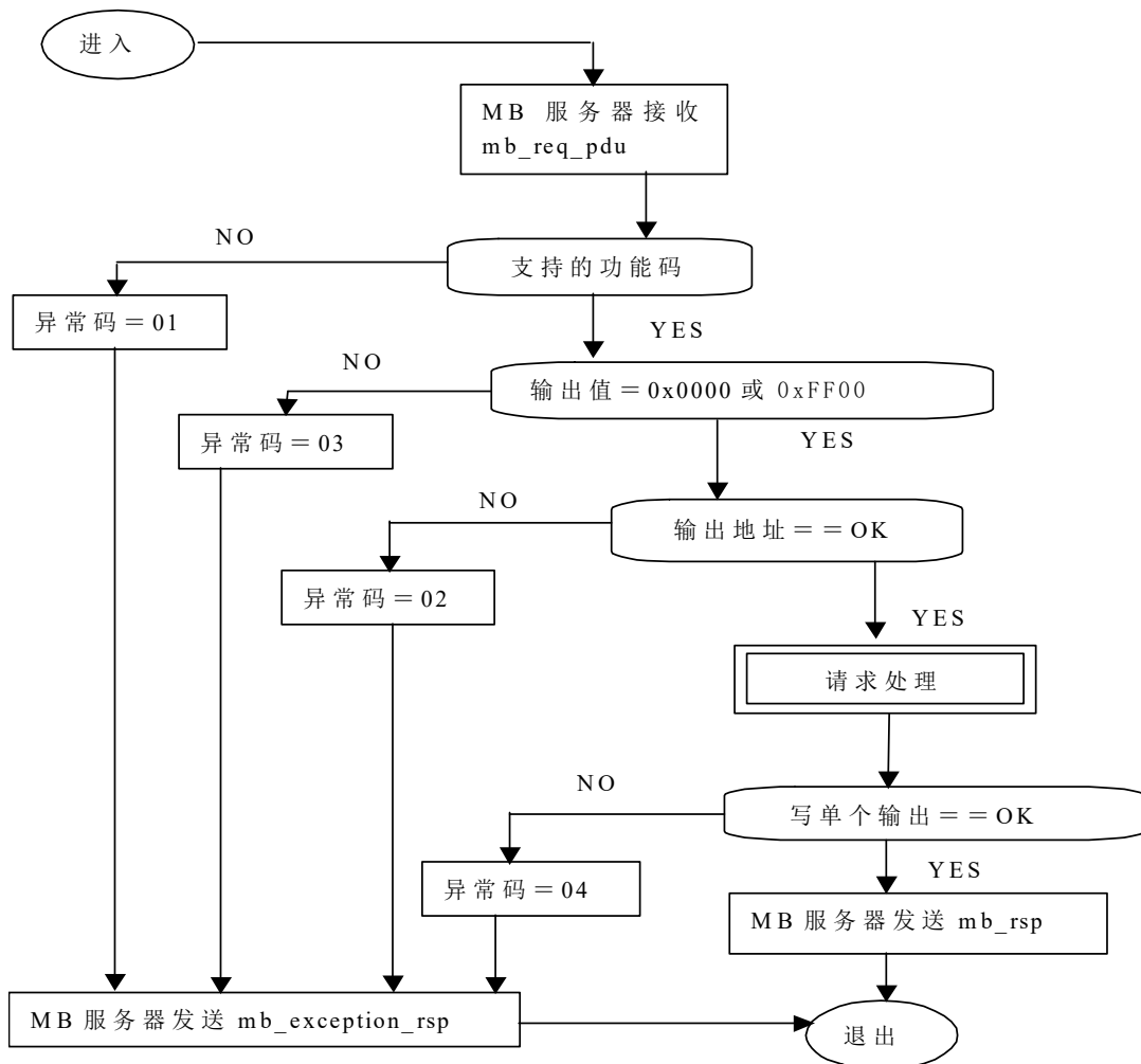
图 22：写单个输出状态图
