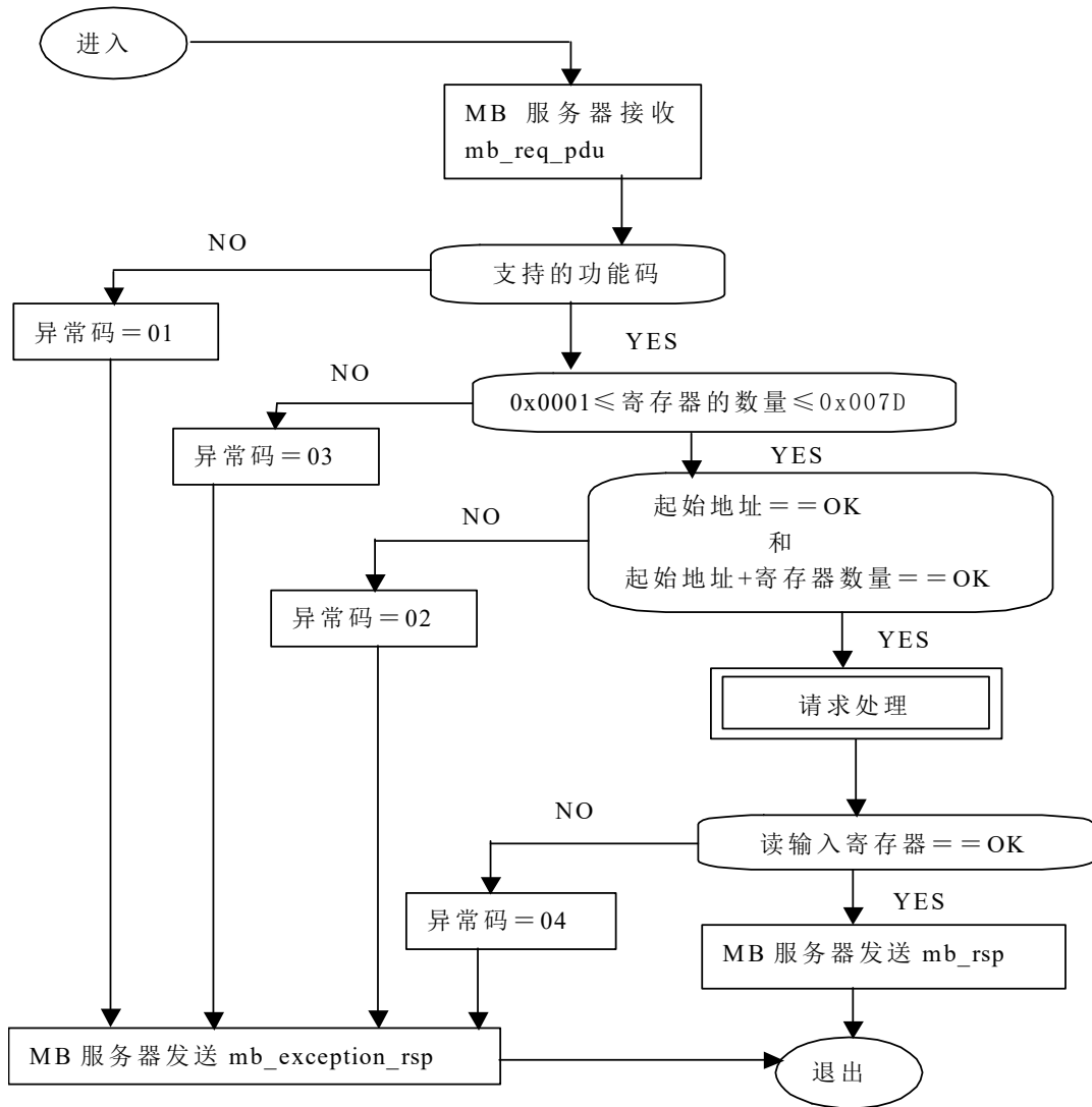
图 21：读输入寄存器的状态图
