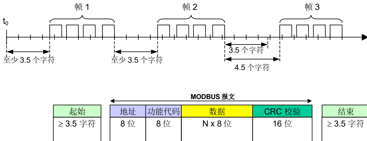
图 10: RTU 报文帧
