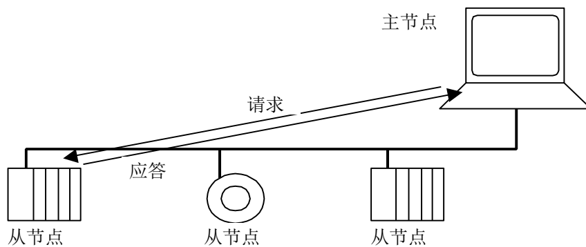
图 3： 单播模式
