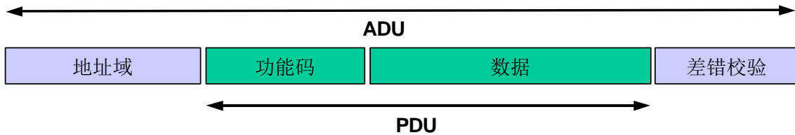
图 12: 通用 MODBUS 帧
