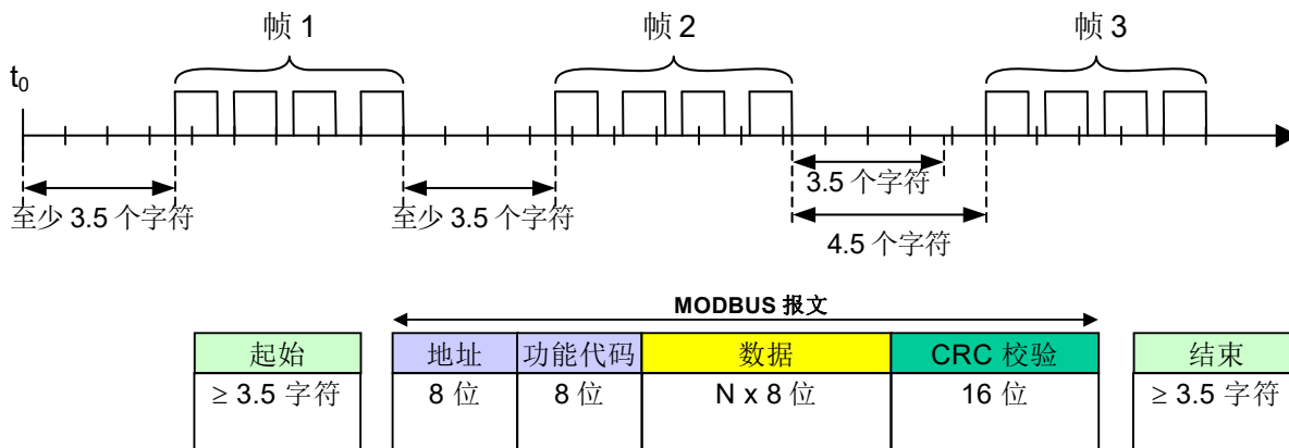
图 1: RTU 报文帧
