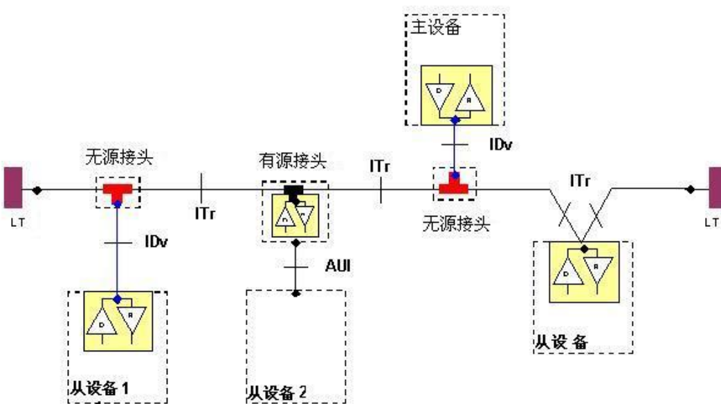
图 1: 串行总线基本结构
