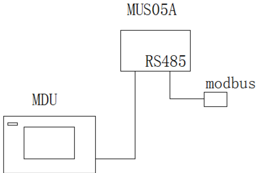
图3-1 接线说明 1
