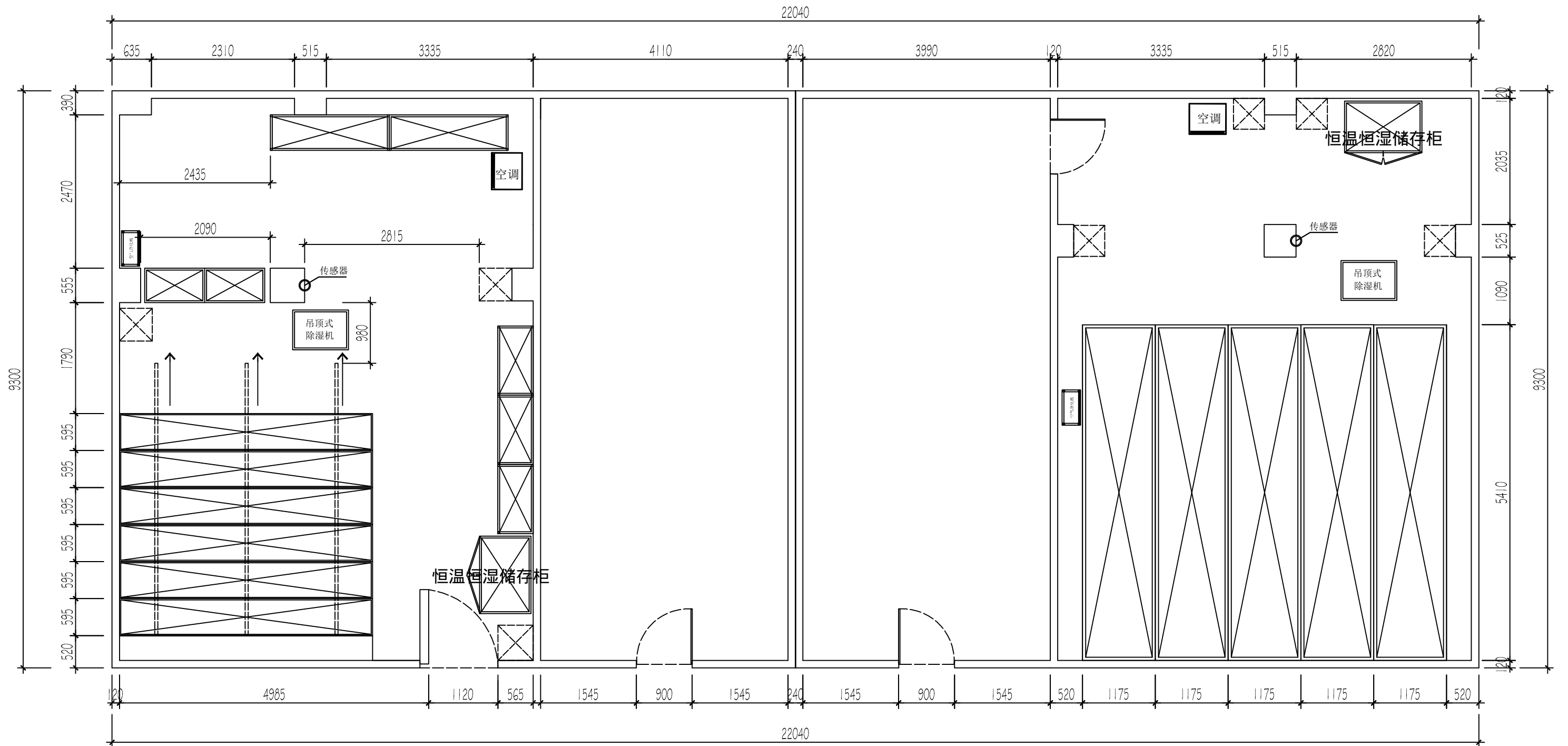
海口市博物馆文物库房调控设备部署示意图
