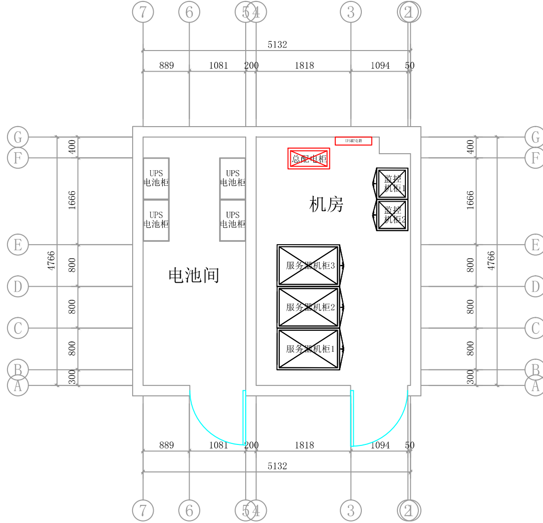
阿拉尔分行机房平面图
