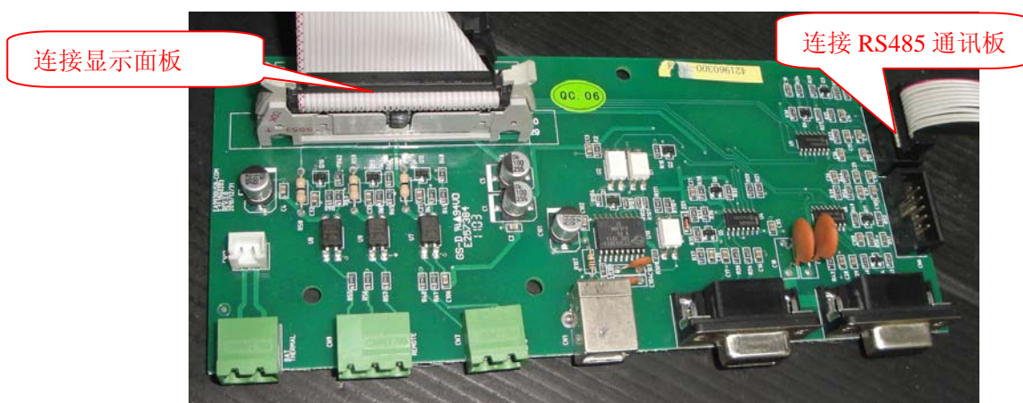
图一 RS232 通讯板
