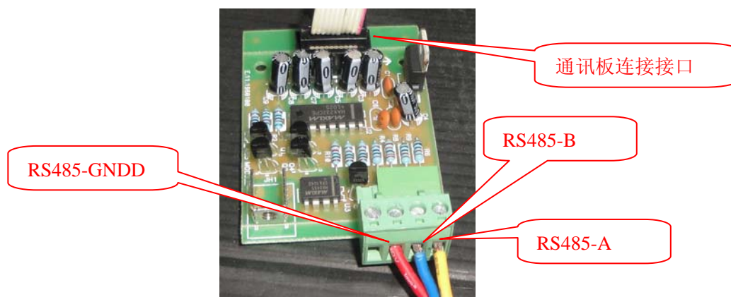
图二 RS485 通讯板
