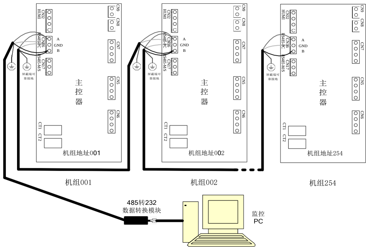
图 1 后台通信系统网络接线图
