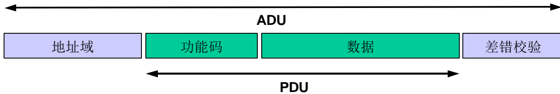
图 12: 通用 MODBUS 帧
