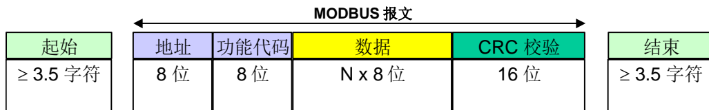
图 1: RTU 报文帧
