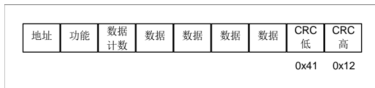
图 26: CRC 字节序列
