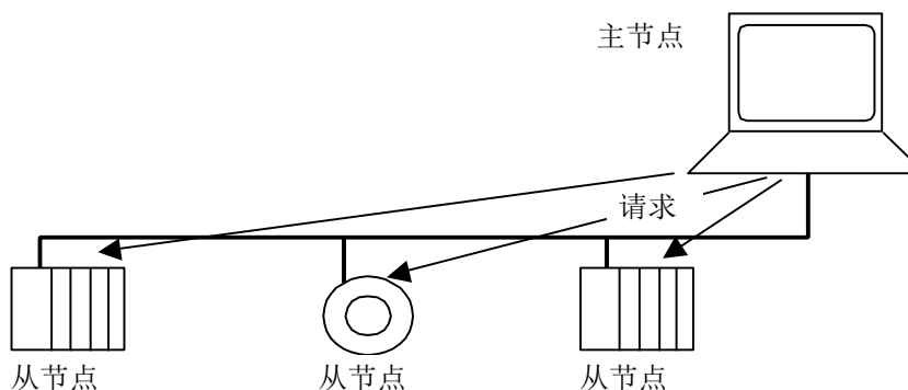
图 4： 广播模式
