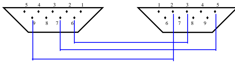
M2502 通讯电缆线
